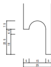
取手断面図 1/1
