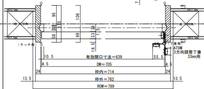
■ラッチ側縦枠
