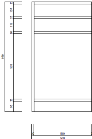
箱枠正面図 1/10
