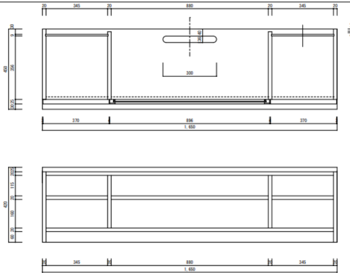
箱枠正面図 1/10 断面図 1/10
