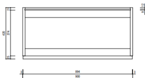
断面図 1/10
