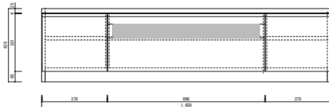
箱枠正面図 1/10 断面図 1/10
