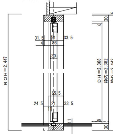
■縦断面図 [4方枠]
