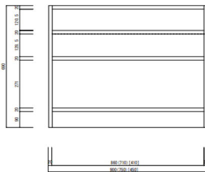
箱枠正面図 1/10
