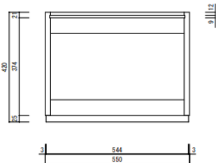
断面図 1/10
