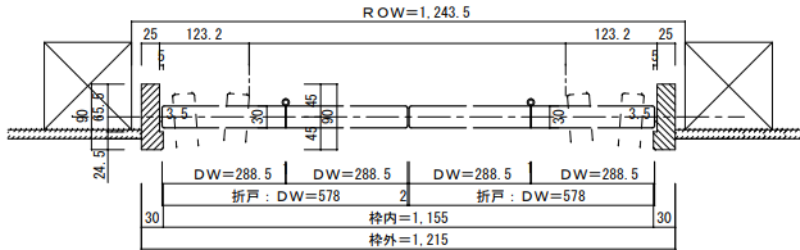
■横断面図
