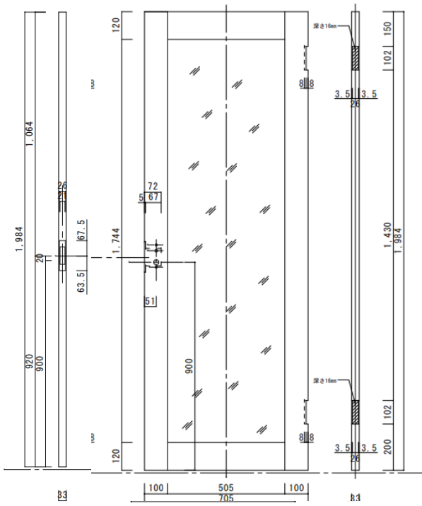
欄間付きドア〔固定枠175巾〕
