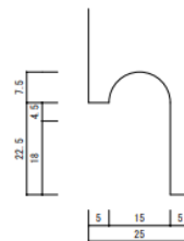
取手断面図 1/1
