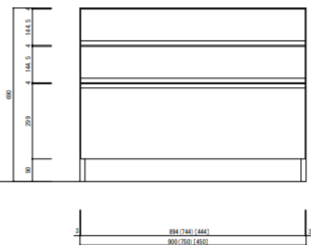
正面図 1/10
