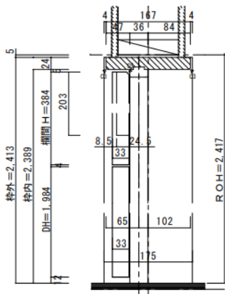
■ 縦断面図
