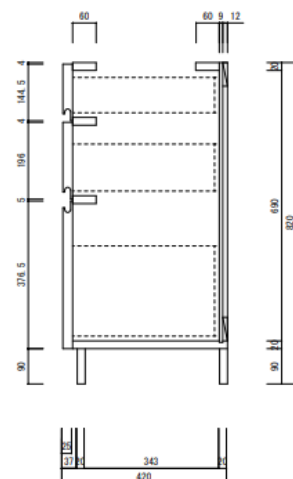
縦断面図 1/10
