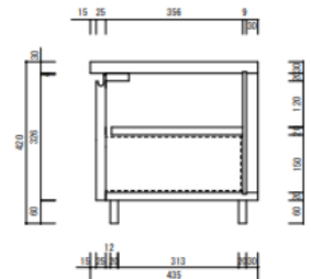
縦断面図 1/10
