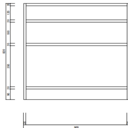
箱枠正面図 1/10
