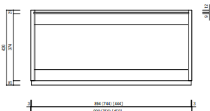
断面図 1/10
