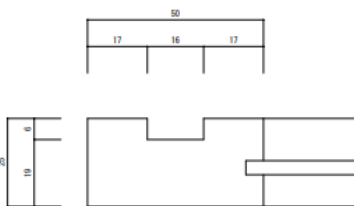
取手堀込横断面 1/1
