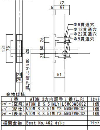
■扉ラッチ側
