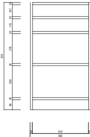
箱枠正面図 1/10
