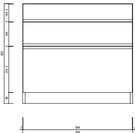
正面図 1/10
