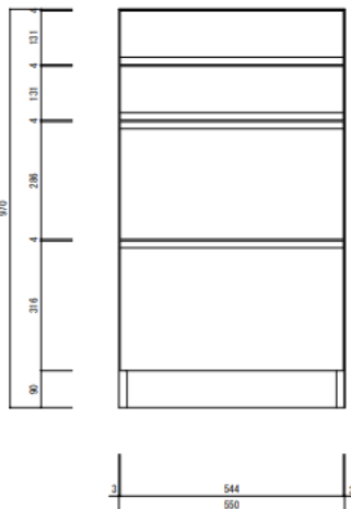
正面図 1/10
