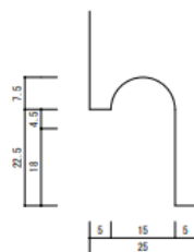
取手断面図 1/1
