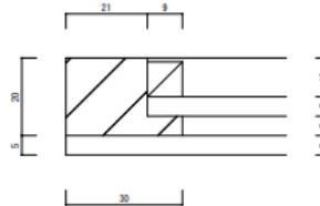
ガラス納め断面図 1/1
