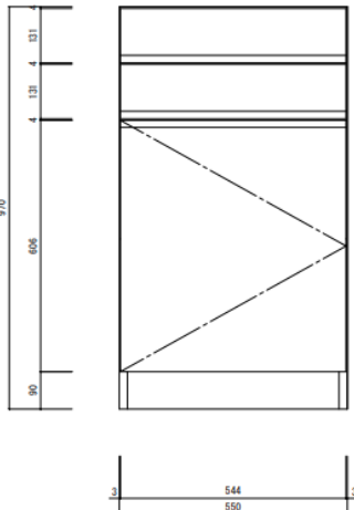
正面図 1/10
