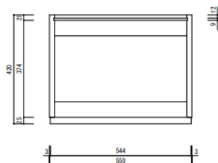
断面図 1/10
