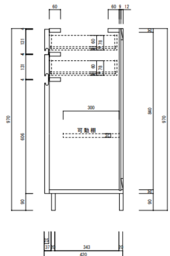
縦断面図 1/10
