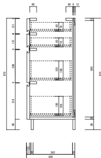
縦断面図 1/10
