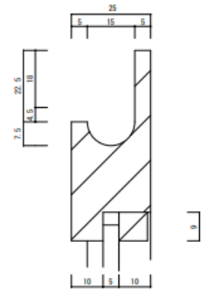
取手断面図 1/1
