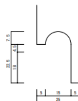
取手断面図 1/1
