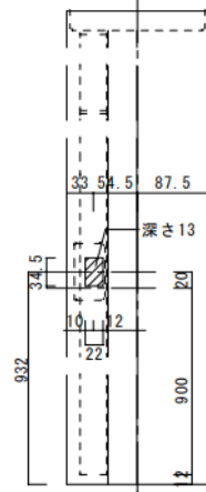
■ラッチ側縦枠
